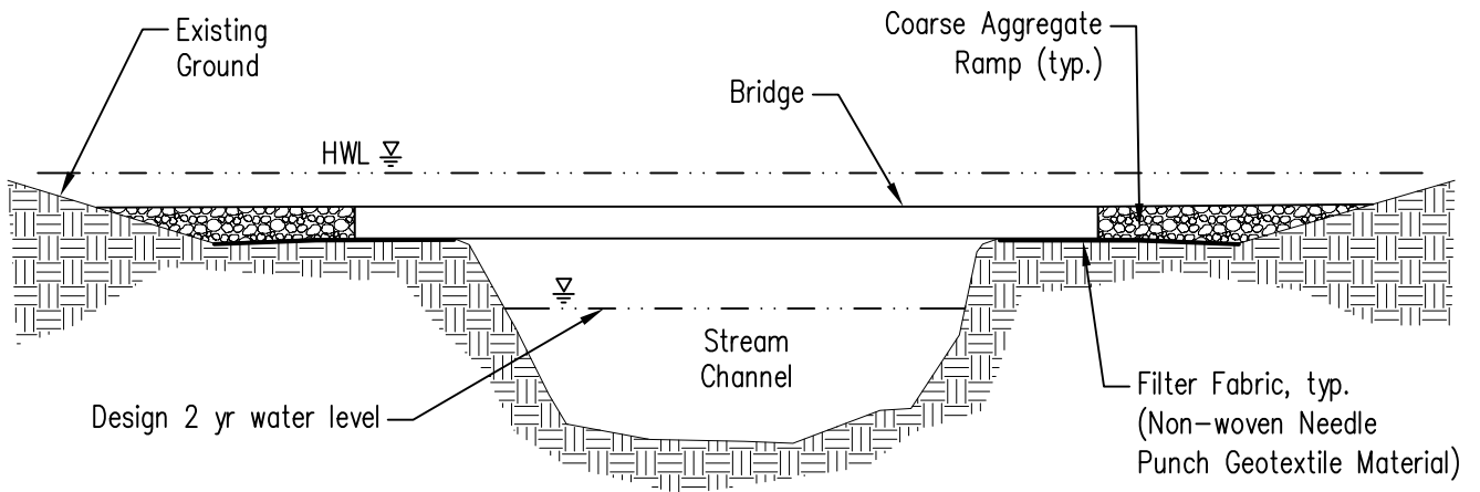
ELEVATION
